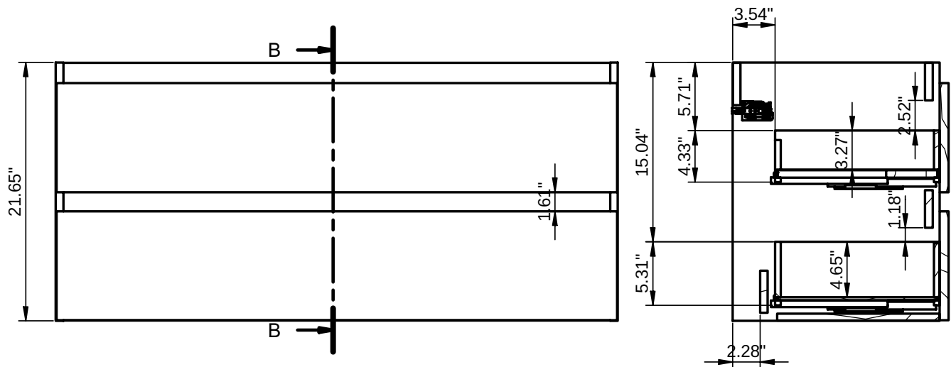
B-B ( 1 : 10 )
