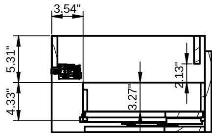
B-B ( 1 : 10 )
