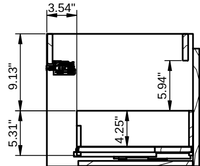
B-B ( 1 : 10 )
