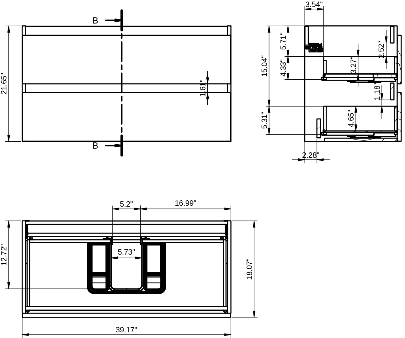
B-B ( 1 : 10 )
