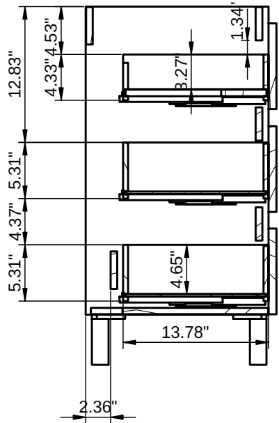
B-B ( 1 : 10 )
