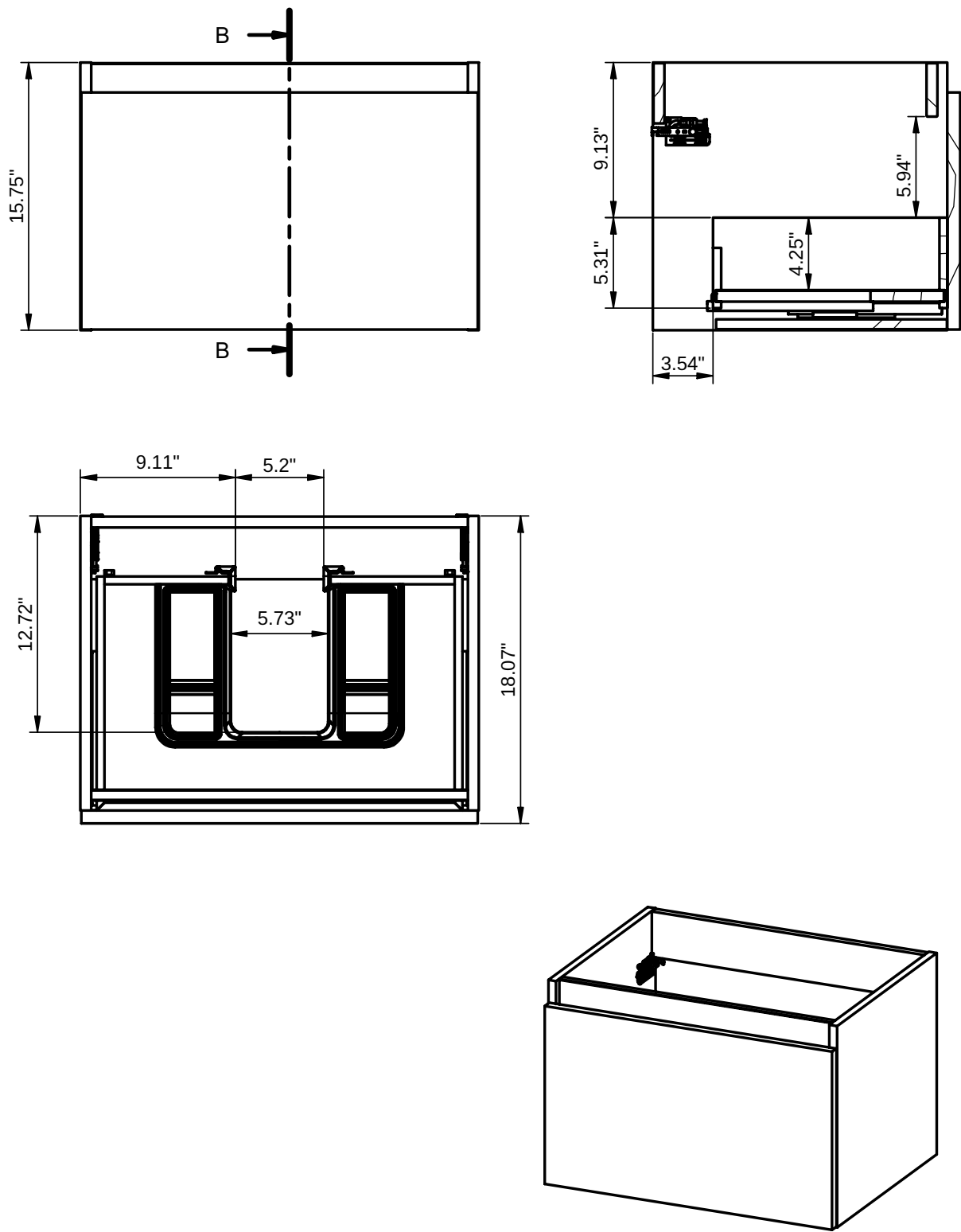
B-B ( 1 : 8 )
