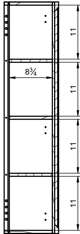
B-B ( 1:10 )
