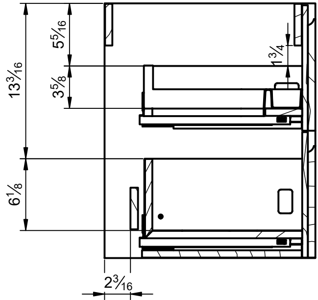
B-B ( 1 : 8 )
